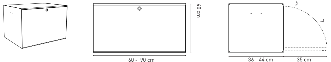
Ribaltina, apertura dall'alto / Hanged tip-up panel, opening from the top
